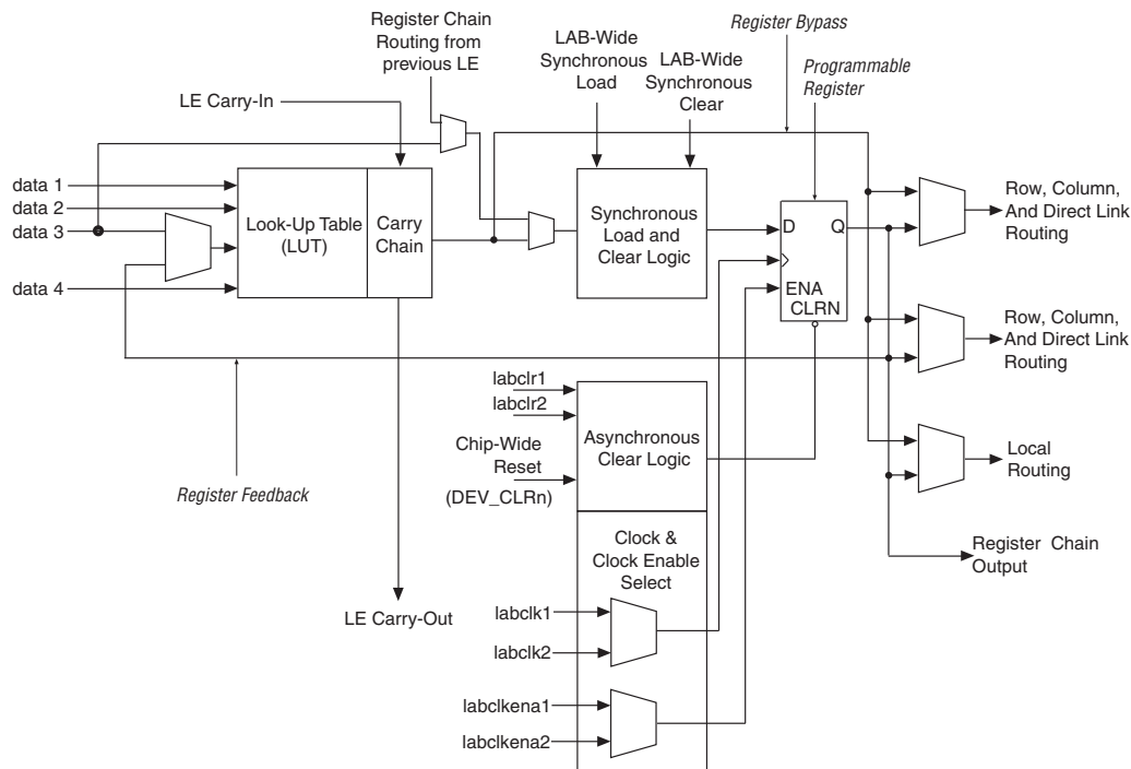
图 2-1. 在 Cyclone IV 器件中的 LE
