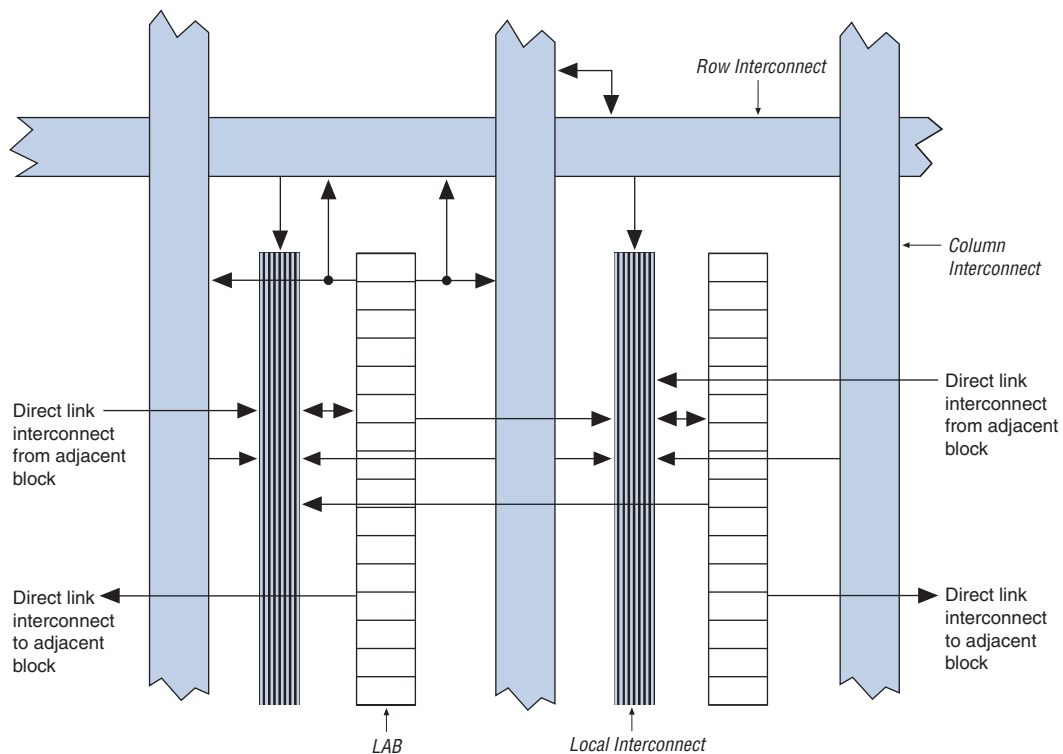
图 2-4. 在 Cyclone IV 器件中的 LAB 结构
