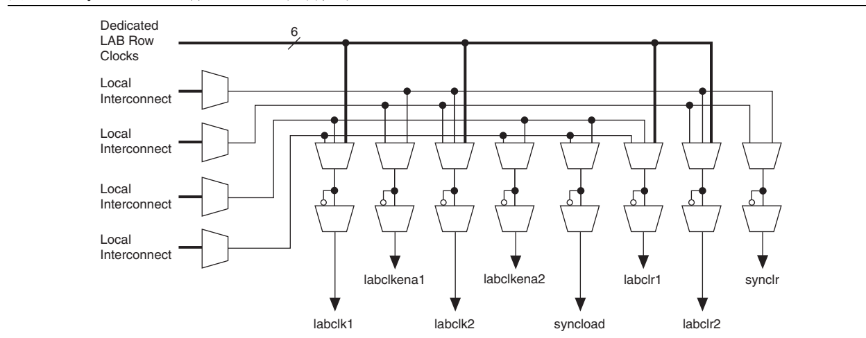
图 2-6. Cyclone IV 器件 LAB-Wide 控制信号
