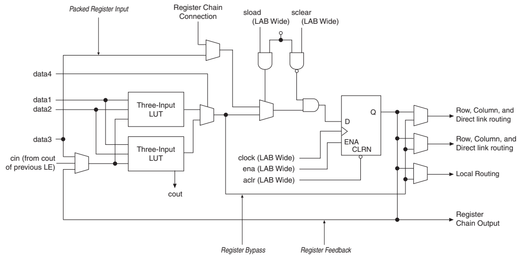
图 2-3. 在 Cyclone IV 器件上算术模式中 LE
